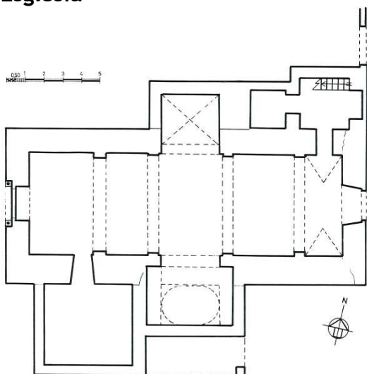
Planta, a escala 1:200, de l'església, amb l'estructura primitiva molt alterada a causa de les reformes que sofrí al llarg de la seva història. J. MARGUÍ-G. ANGLADA
